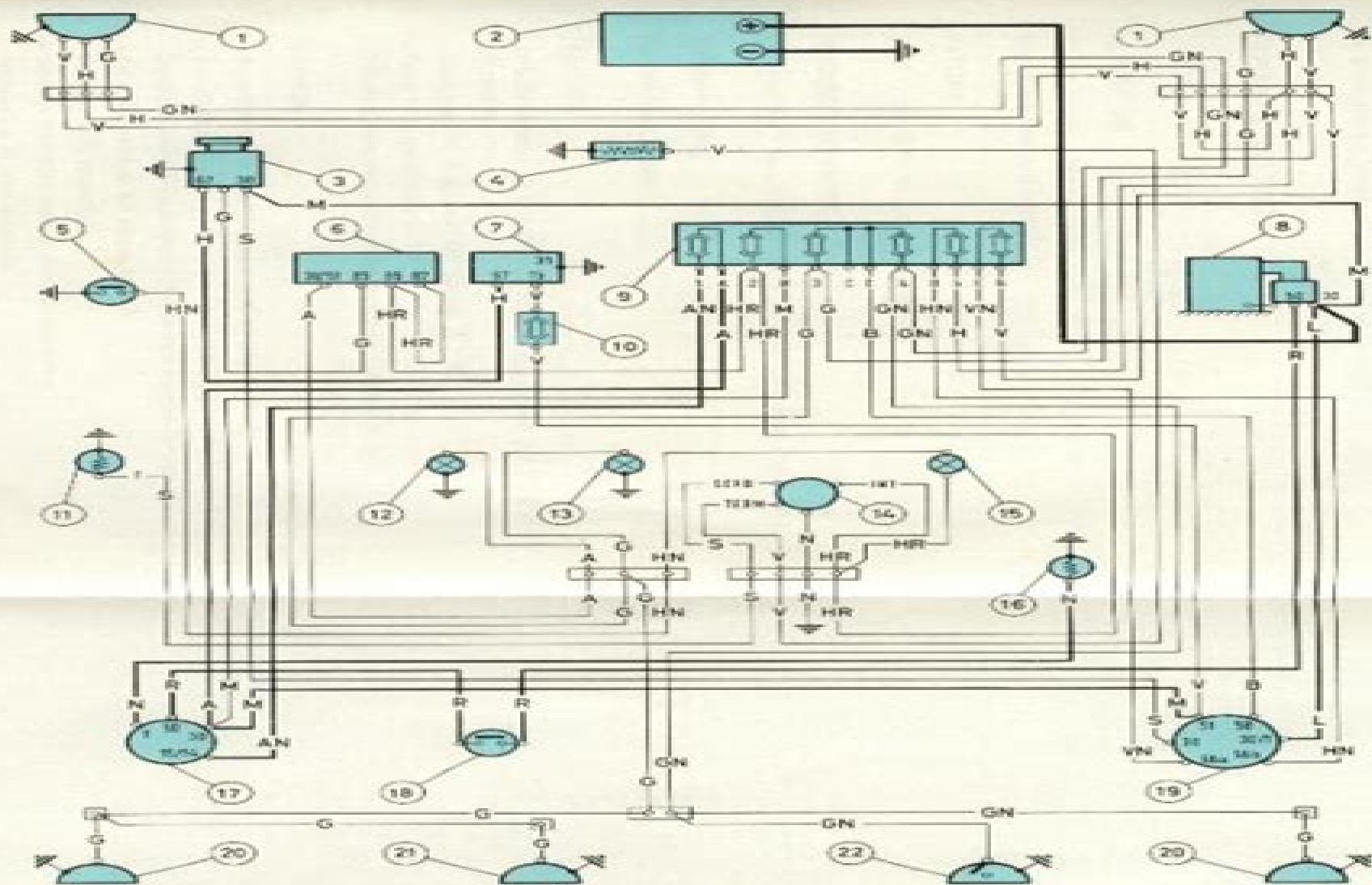
Fig. 22. - Schema dell'impianto elettrico (tensione 12 V).
