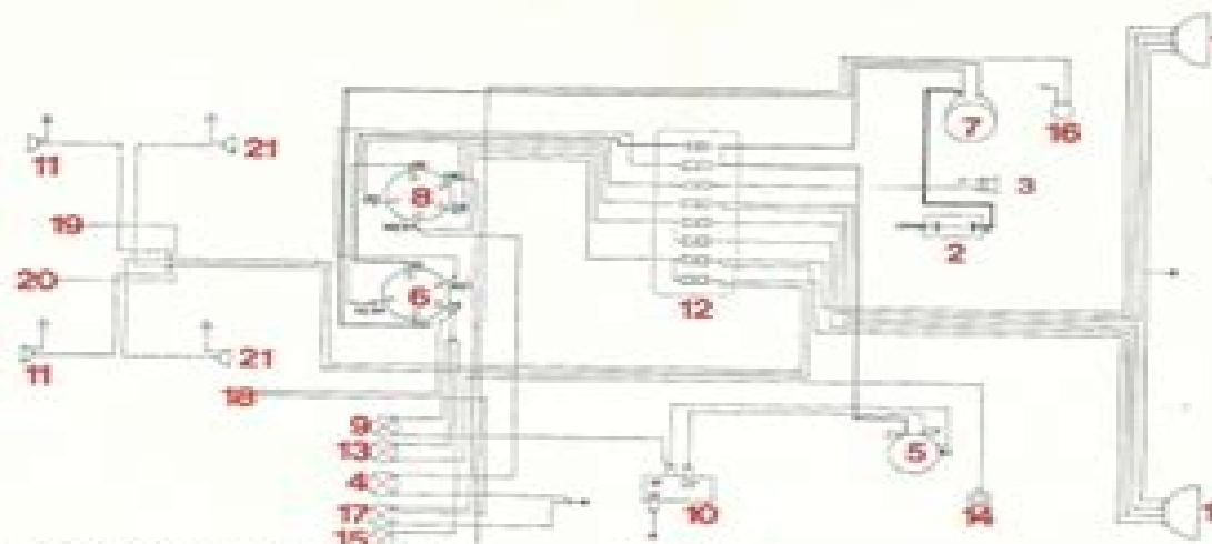
Fig. 21 - Schéma de l'installation électrique
