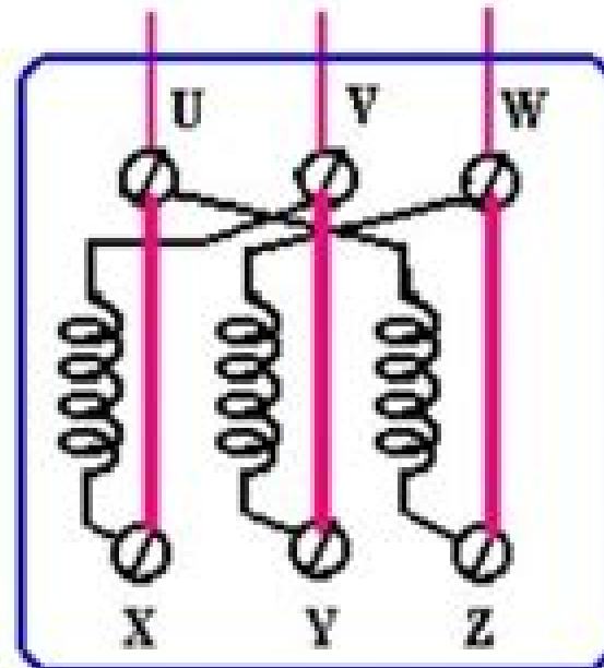
COLLEGAMENTO A TRIANGOLO
