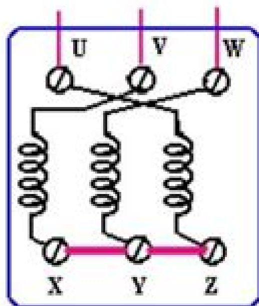
COLLEGAMENTO A STELLA
