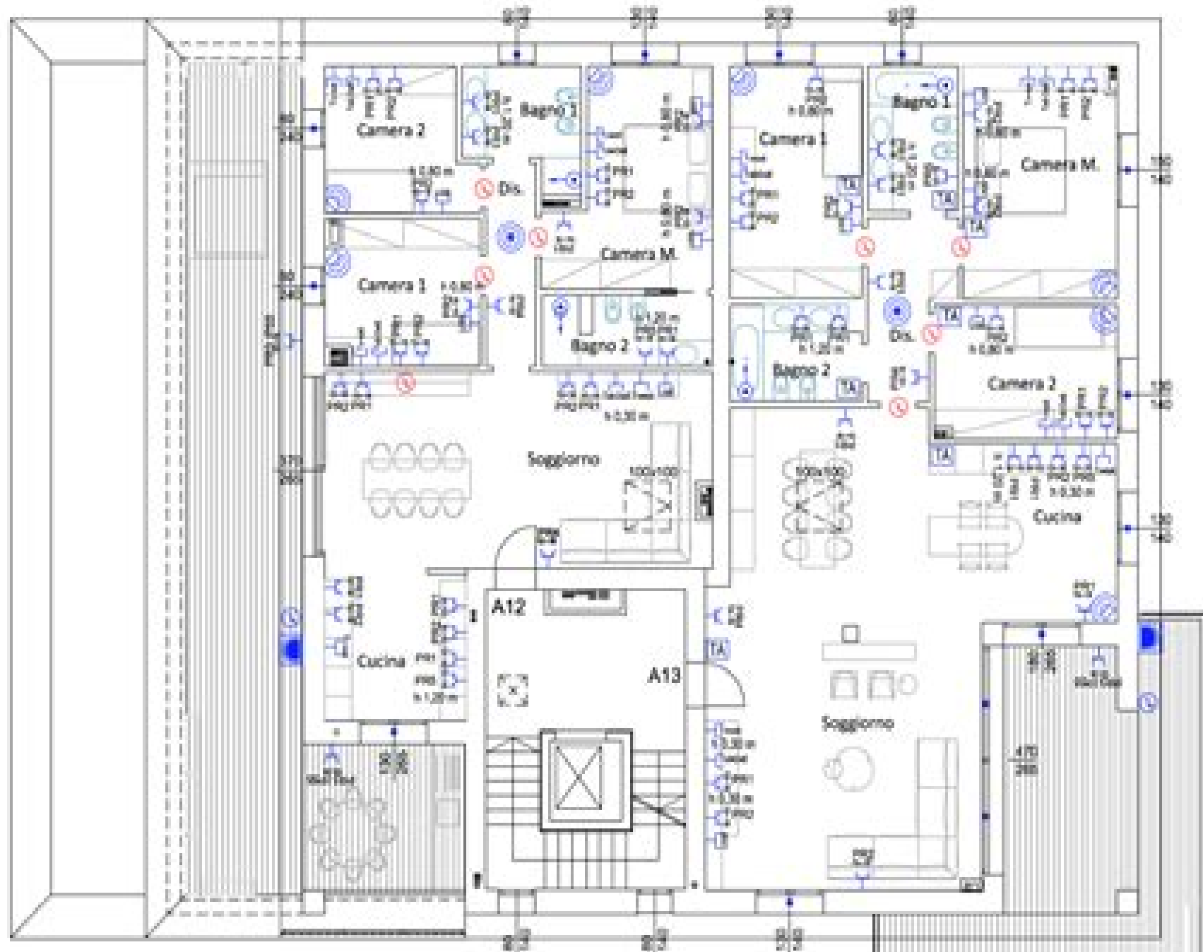
Pianta piano 4°
