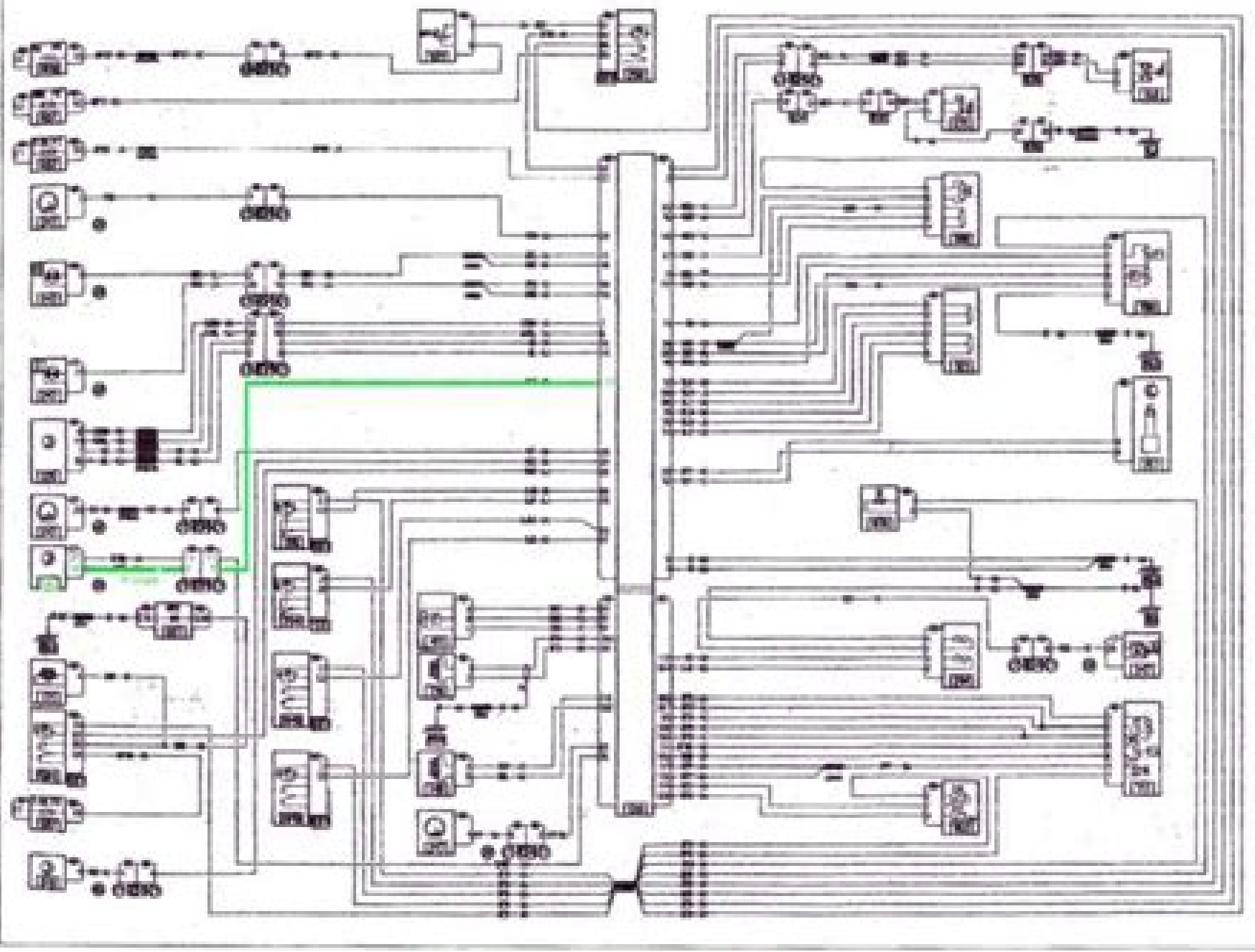
ESQUEMA DE CONEXIÓN DE LA CENTRAL DE CONTROL DE LA PLANTA
