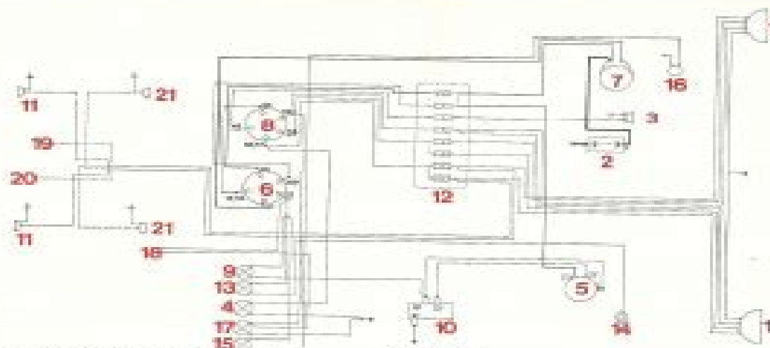
Fig. 55 - Schéma de l'installation électrique
