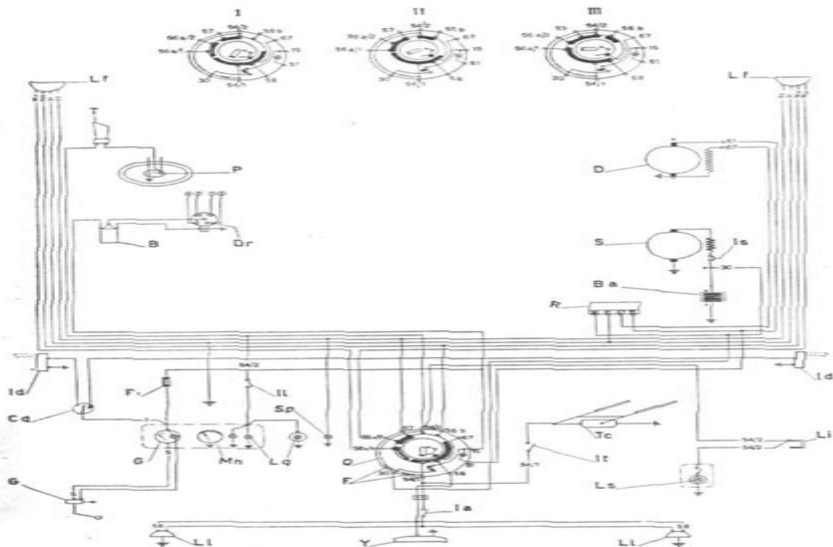
Fig. 54. - Schema dell'impianto elettrico.
