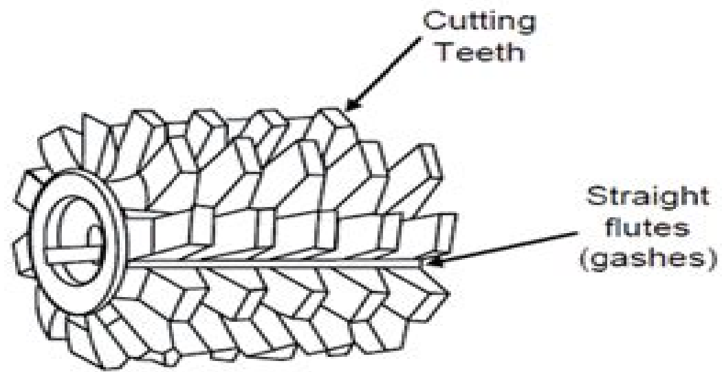
Gear Hob
