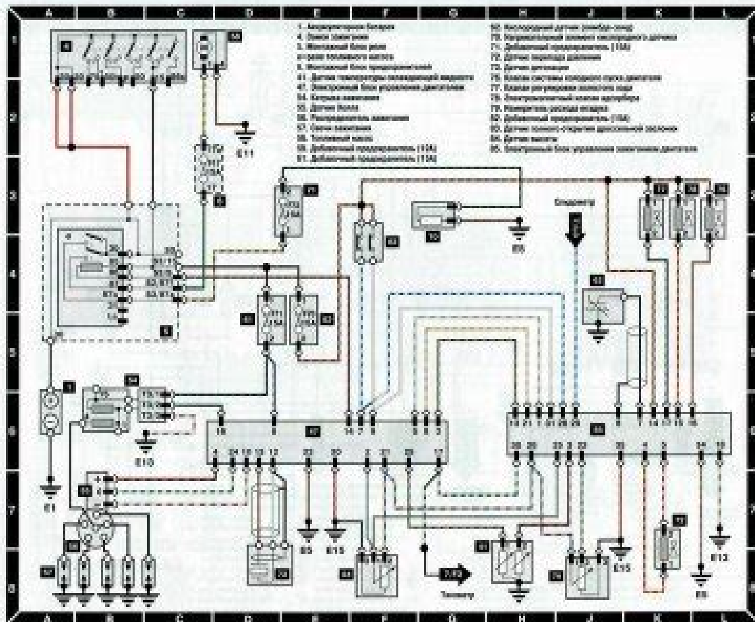
Схема 10. Система управления двигателем VAZ-100
