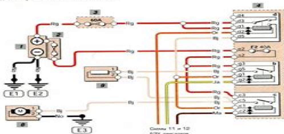
Вентилятор системы охлаждения двигателя
