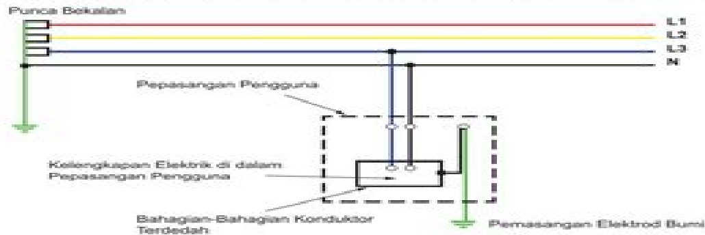
Rajah 5.1: Contoh Sistem TT (Fasa Tunggal)
