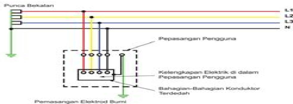
Rajah 5.2: Contoh Sistem TT (Fasa Tiga)
