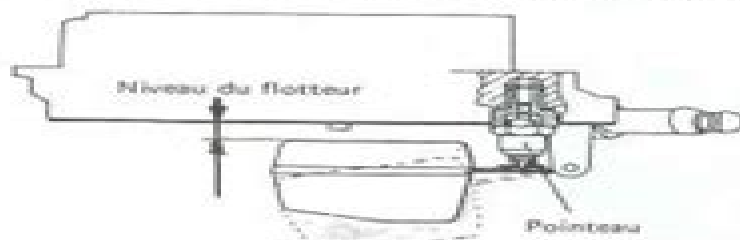
Carburateur Weber 32 DMTR : Niveau de core
