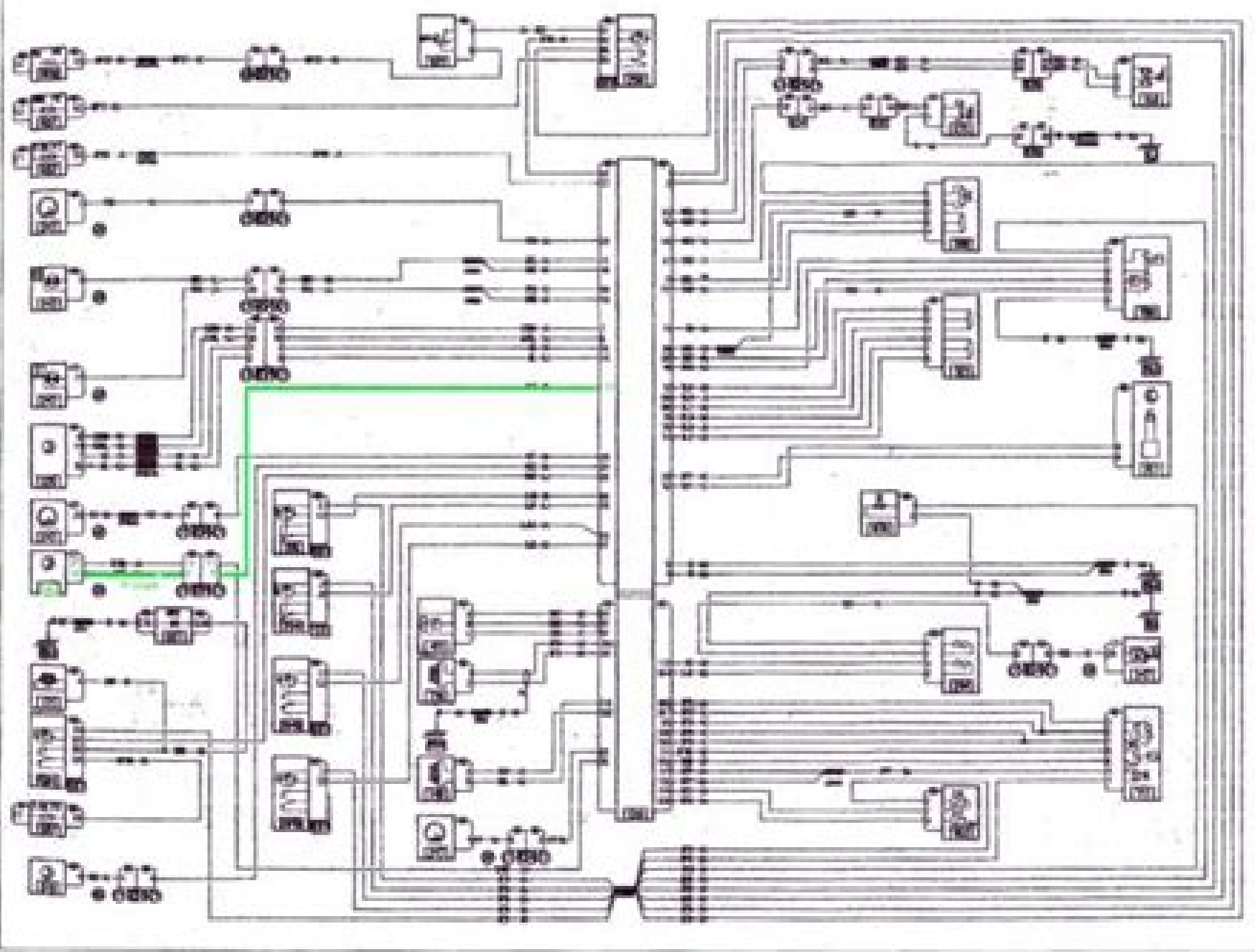
ESQUEMA DE CONEXIÓN DE LA CENTRAL DE CONTROL (PANTALLA 250.145)
