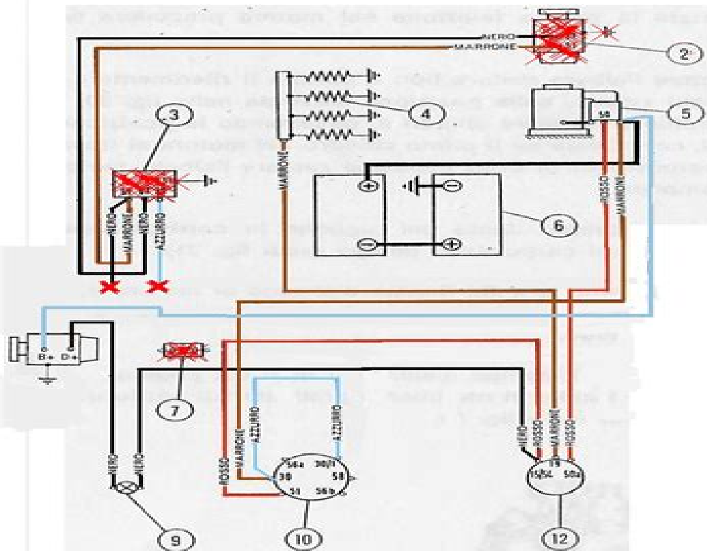
Fig. 34. - Schema dell'impianto elettrico (tensione 24 volt).
