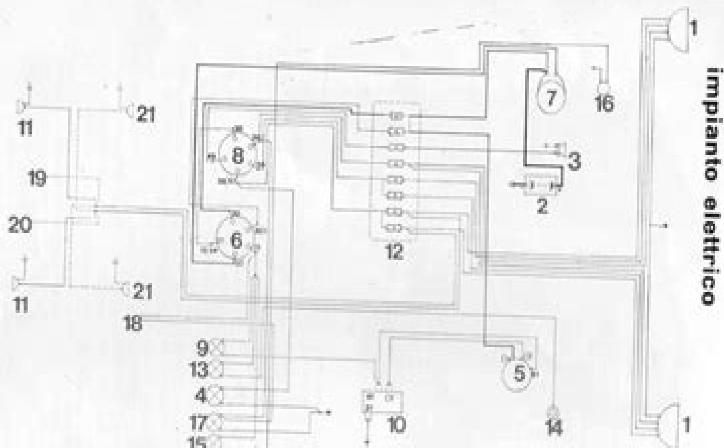
fig. 25 Schema impianto elettrico
