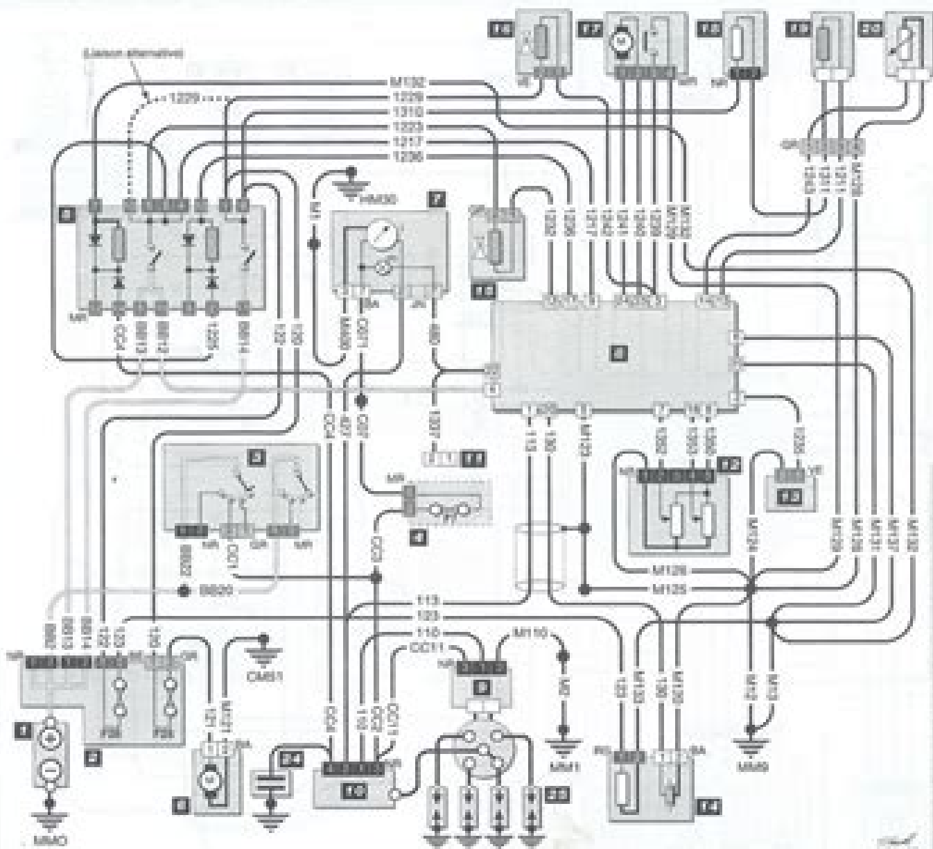
Schéma 14 : Injection-allumage (système Bosch A2.2) et compte-tours sur moteurs TU1ML et TU3MZ - à partir du n° de châssis 55 191 756
