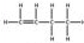
BUT-1-ENE
