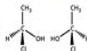
L: (S)-1-CHLOROETHANOL R: (R)-1-CHLOROETHANOL
