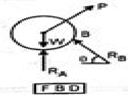
l) Wheel of wt. W
